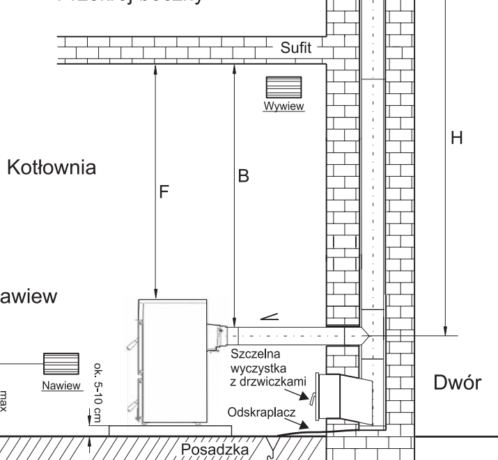
Przekrój boczny
