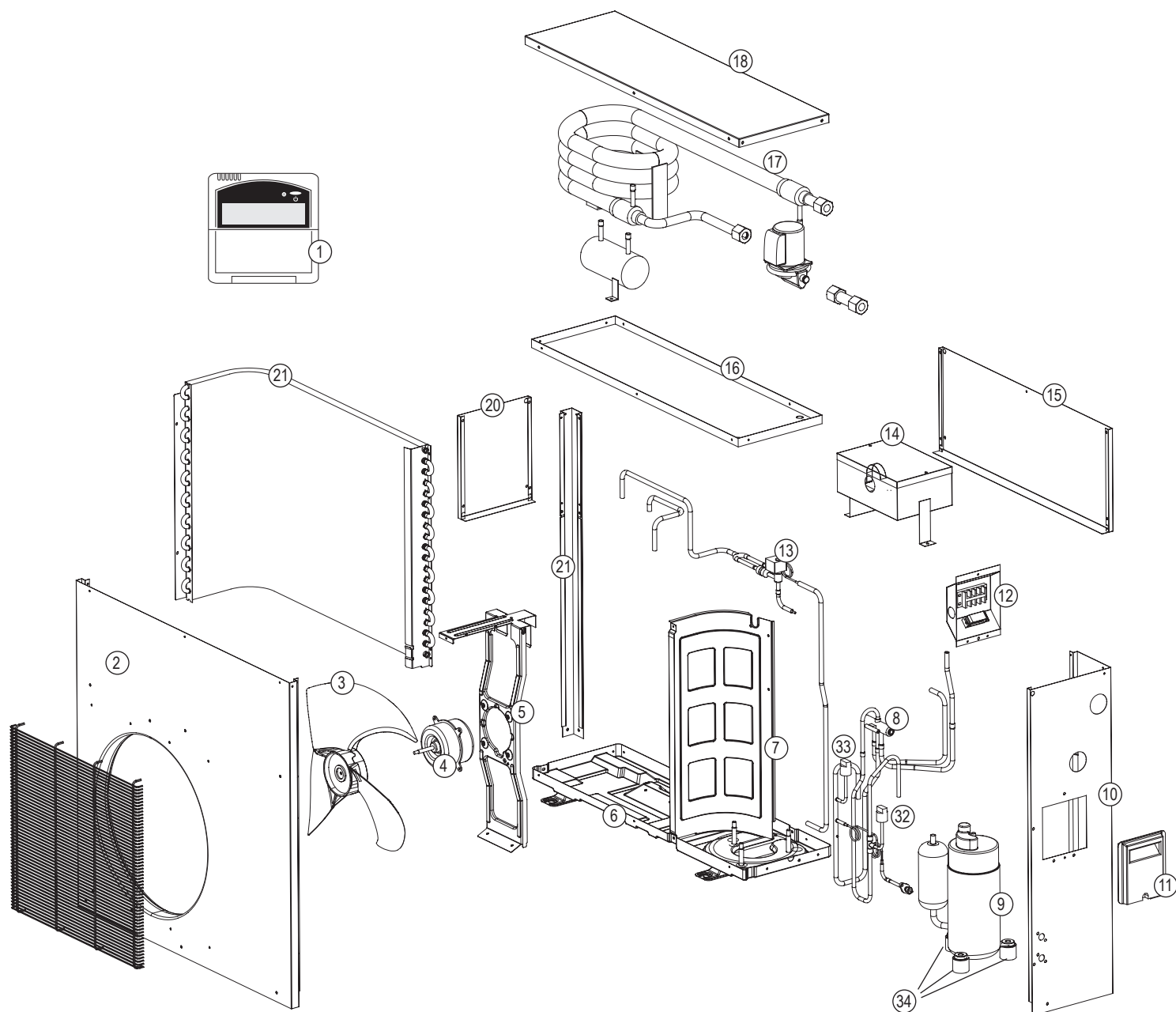
Rys. Rysunek rozstrzelony pompy ciepła powietrze-woda HITPump WASSER.
