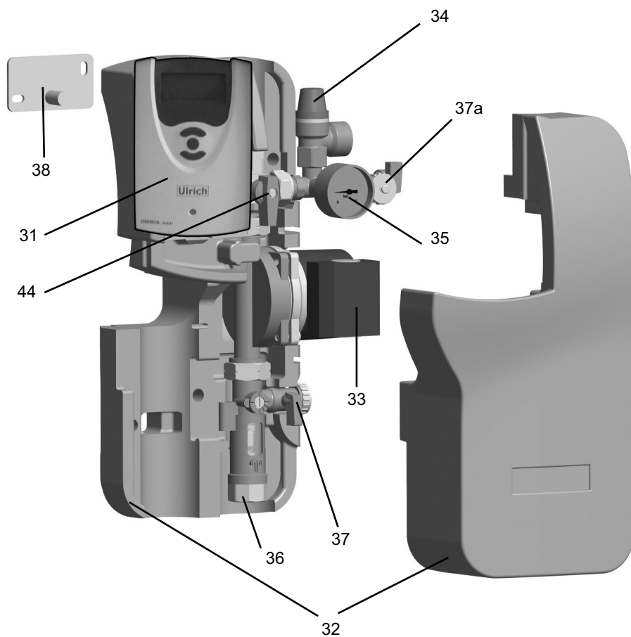
Rys. nr 3. Rysunek budowy grupy hydraulicznej typ III.
