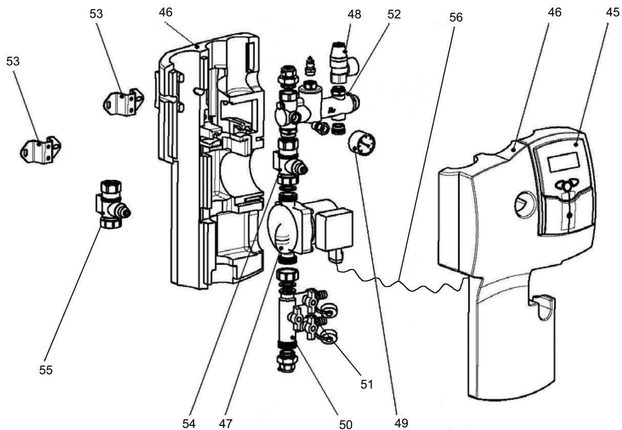
Rys. nr 4. Rysunek budowy grupy hydraulicznej typ IV.
