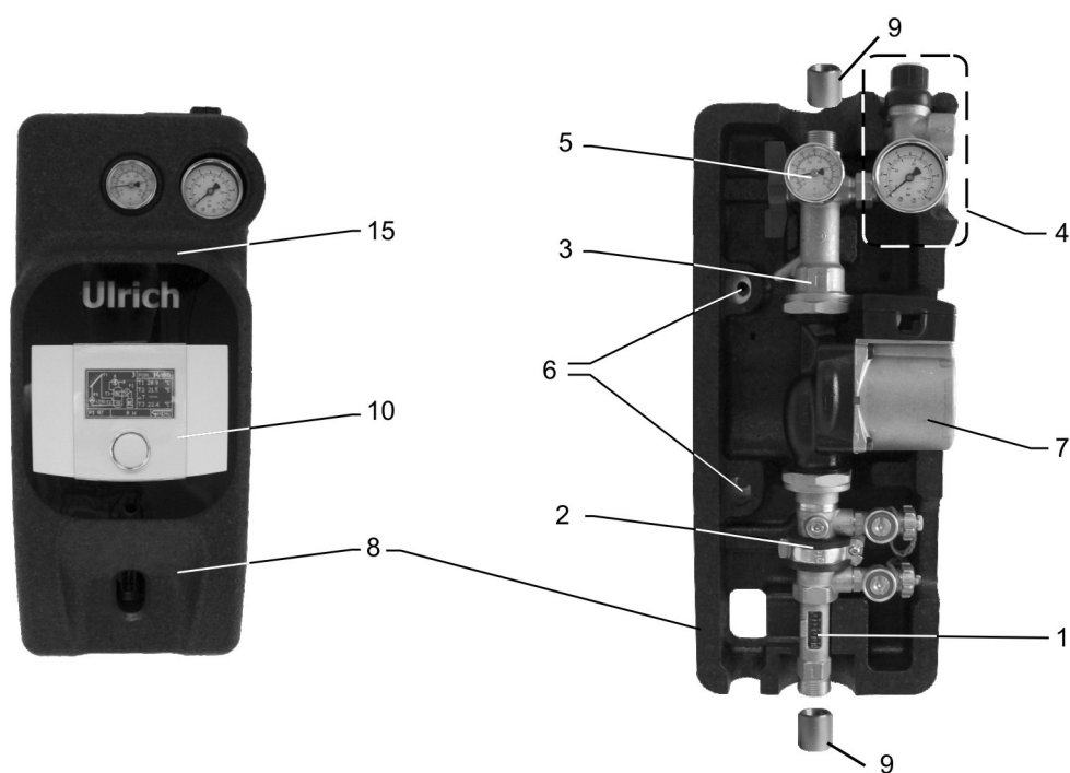
Rys. nr 1. Rysunek budowy grupy hydraulicznej typ I.
