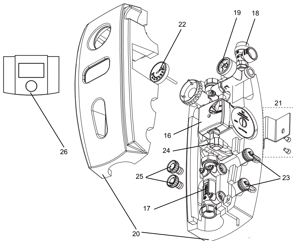
Rys. nr 2. Rysunek budowy grupy hydraulicznej typ II.
